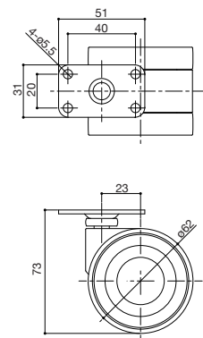
DF1-0MP-ZN2-062 平付けタイプ Plate stem type
